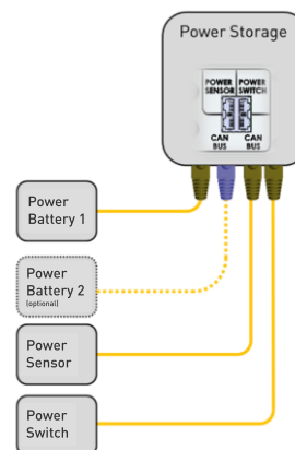
Zusätzliche Power Switch und Power Sensor Kommunikation
