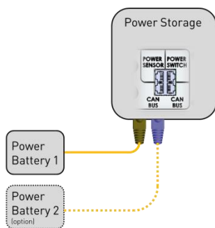
Standard Kommunikation mit der Power Batterie
