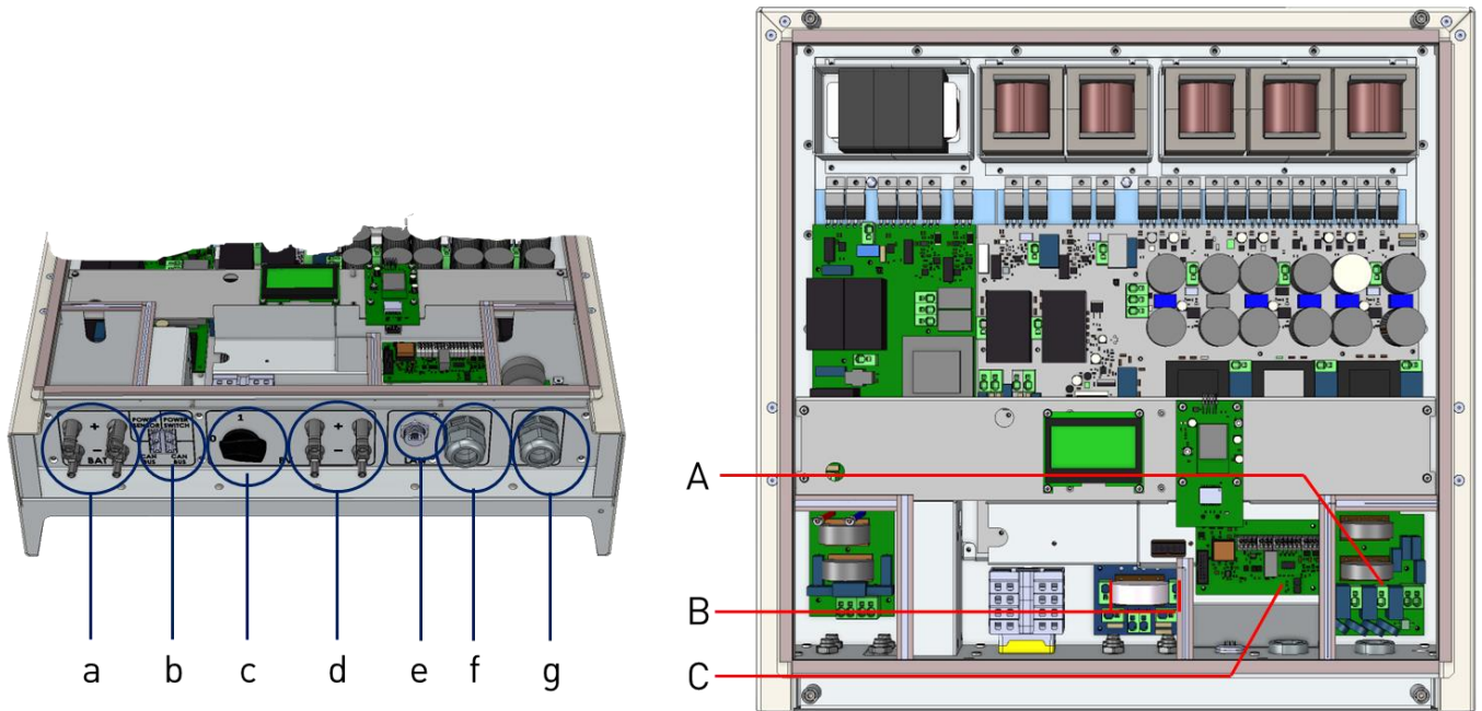
Abb. 5-1 Übersicht Anschlußbereich und innere Verbindungsteile
